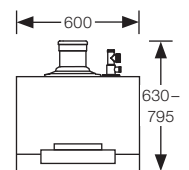
Logano plus KBH192i
